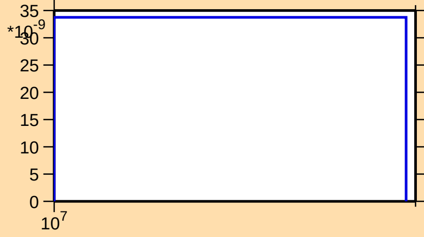
\sigma vs. E for ^{107}\text{Sn}(\text{mt } 45)
