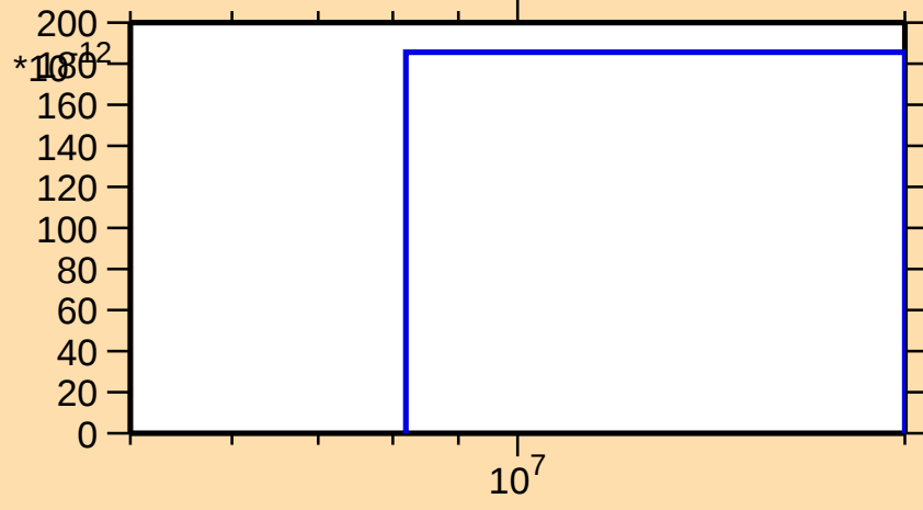
\sigma vs. E for ^{107}\text{Sn}(\text{mt } 34)
