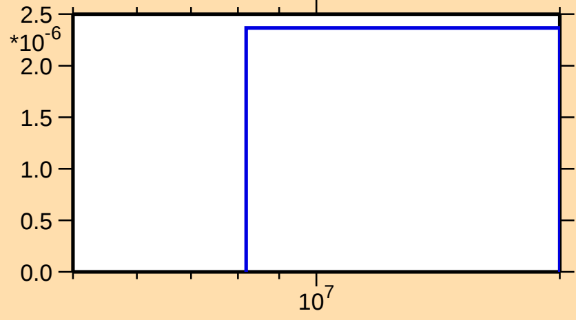
\sigma vs. E for ^{166}\text{Ta}(\text{mt } 45)
