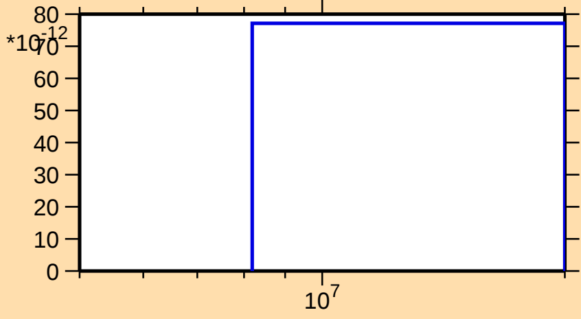
\sigma vs. E for ^{166}\text{Ta}(\text{mt } 34)
