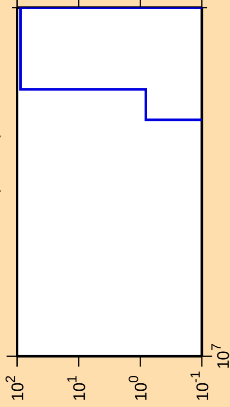
\Delta\sigma/\sigma vs. E for ^{167}\text{Ta}(\text{mt } 34)
