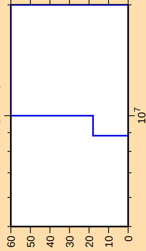
\Delta\sigma/\sigma vs. E for ^{167}\text{Ta}(\text{mt } 45)
