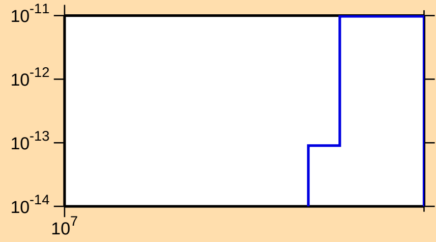
\sigma vs. E for ^{167}\text{Ta}(\text{mt } 34)
