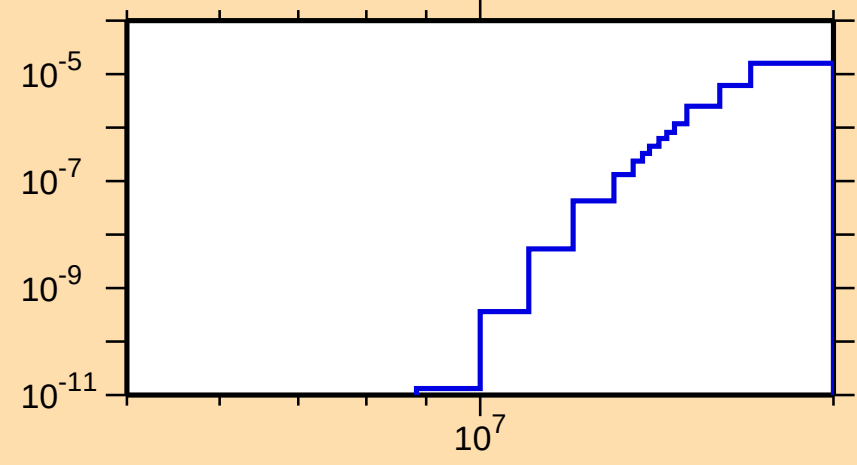
\sigma vs. E for ^{167}\text{Ta}(\text{mt } 45)
