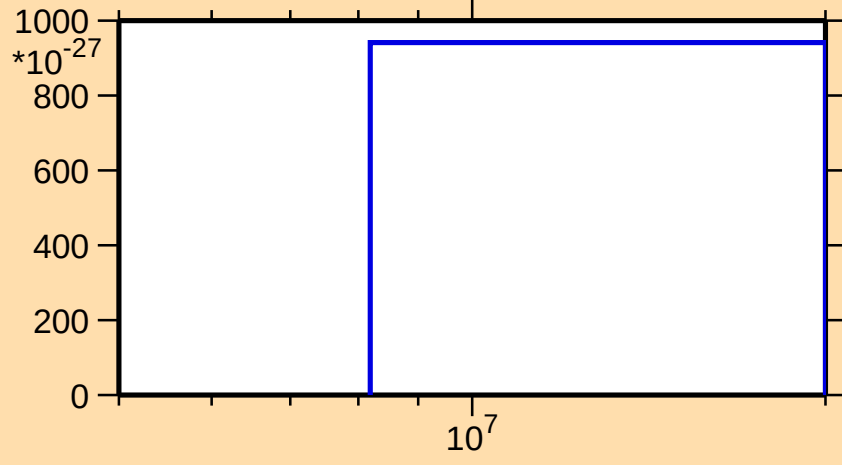
\sigma vs. E for ^{183}\text{Ta}(\text{mt } 42)
