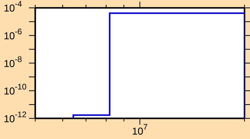
\sigma vs. E for ^{114}\text{Xe}(\text{mt } 45)
