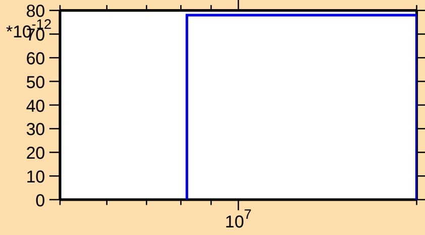
\sigma vs. E for ^{114}\text{Xe}(\text{mt } 34)
