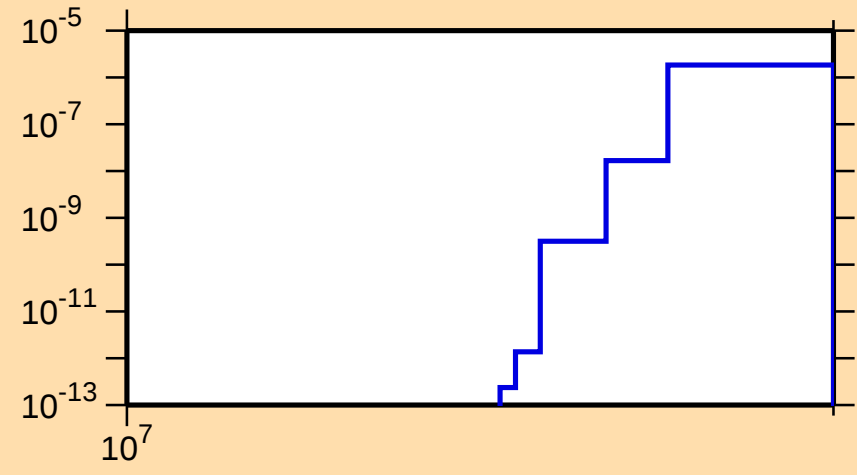
\sigma vs. E for ^{61}\text{Zn}(\text{mt } 45)
