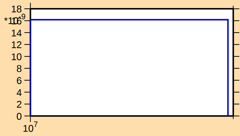
\sigma vs. E for ^{61}\text{Zn}(\text{mt } 45)
