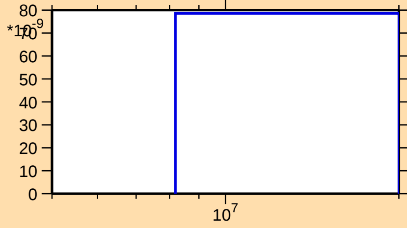
\sigma vs. E for ^{61}\text{Zn}(\text{mt } 34)
