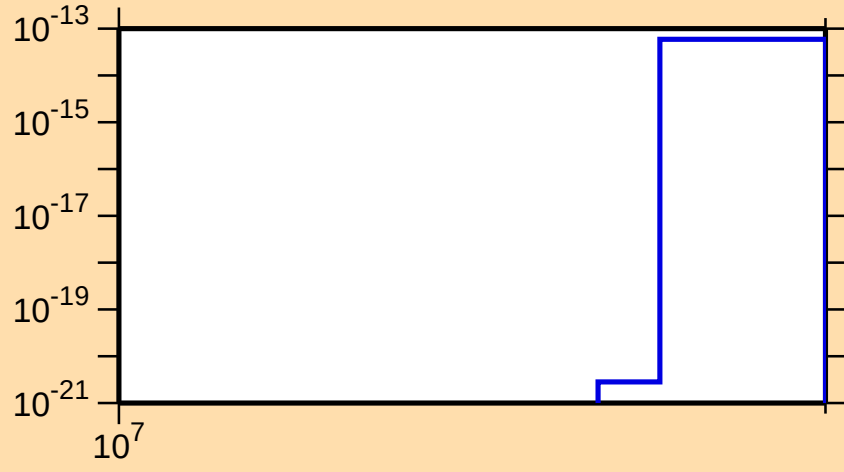
\sigma vs. E for ^{248}\text{Es} (mt 42)
