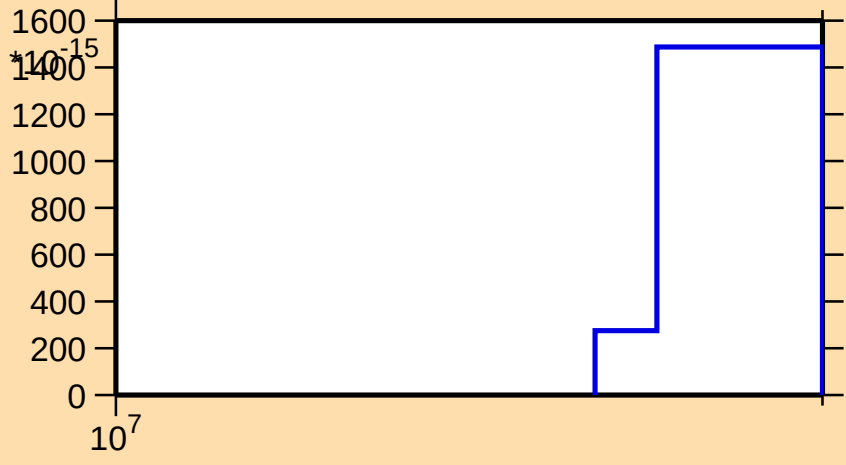
\sigma vs. E for ^{248}\text{Es}(\text{mt } 45)
