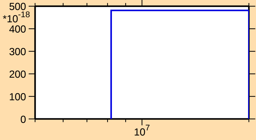
\sigma vs. E for ^{248}\text{Es}(\text{mt } 42)
