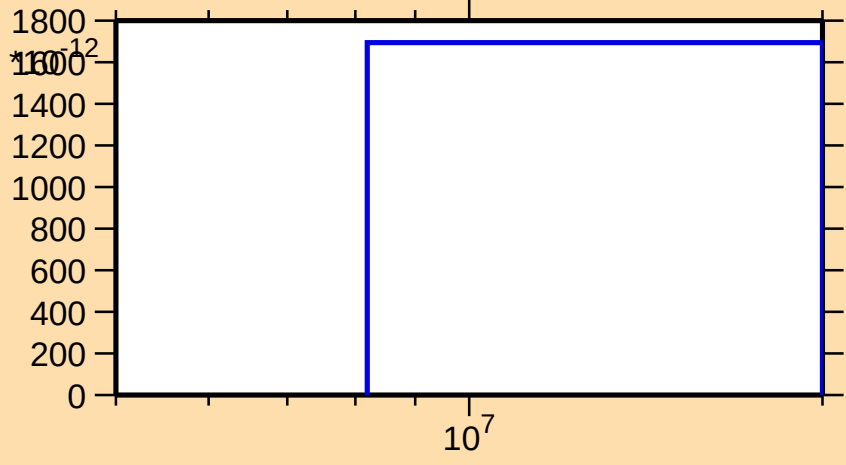
\sigma vs. E for ^{139}\text{Gd}(\text{mt } 34)
