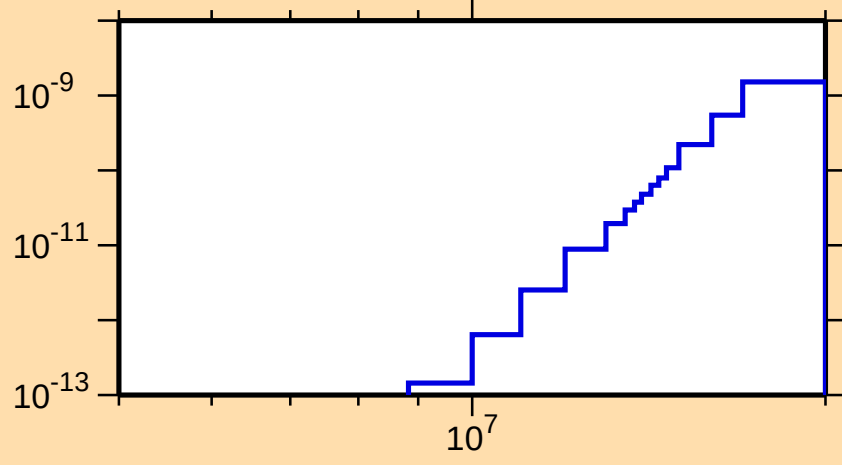
\sigma vs. E for ^{254}\text{Lw(mt 45)}
