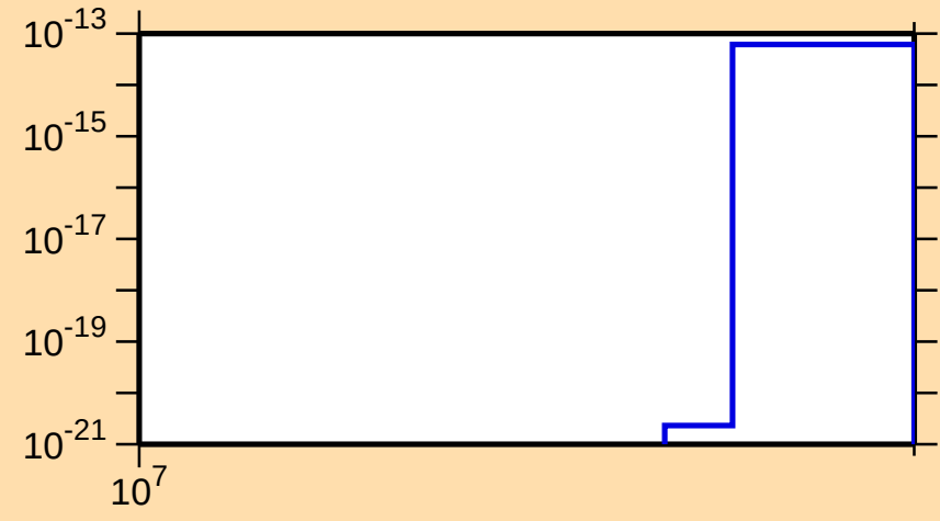
\sigma vs. E for ^{254}\text{Lw}(\text{mt } 42)
