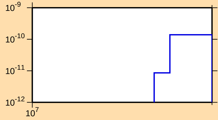
\sigma vs. E for ^{254}\text{Lw}(\text{mt } 34)
