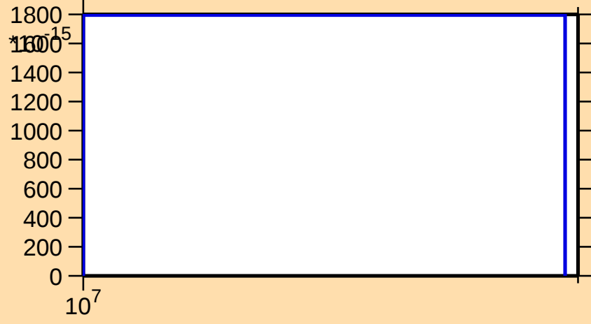
\sigma vs. E for ^{254}\text{Lw(mt 34)}
