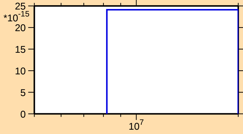
\sigma vs. E for ^{147}\text{Sm}(\text{mt } 34)
