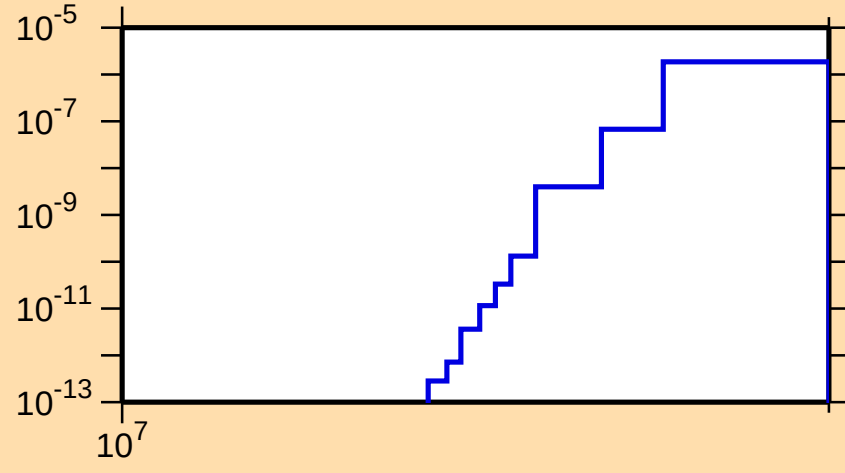
\sigma vs. E for ^{86}\text{Nb}(\text{mt } 45)
