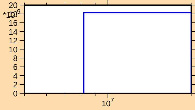
\sigma vs. E for ^{86}\text{Nb}(\text{mt } 45)
