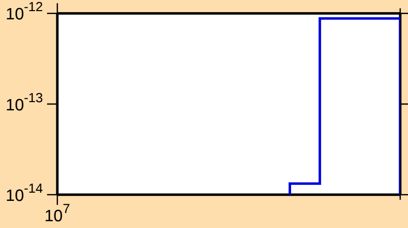
\sigma vs. E for ^{257}\text{No}(\text{mt } 34)
