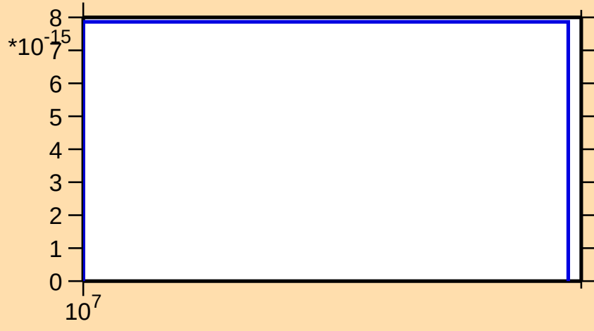
\sigma vs. E for ^{257}\text{No}(\text{mt } 34)
